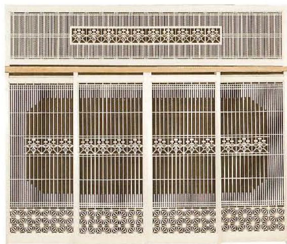
▼FM-668 (WS-124) 八角面桐之葉帯腰麻之葉 (WR-116) 吹寄額桐之葉
