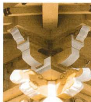
三斗組 (みつとぐみ)
